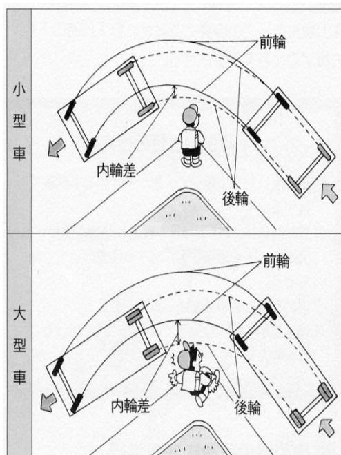
【小型車と大型車の内輪差の違い】
